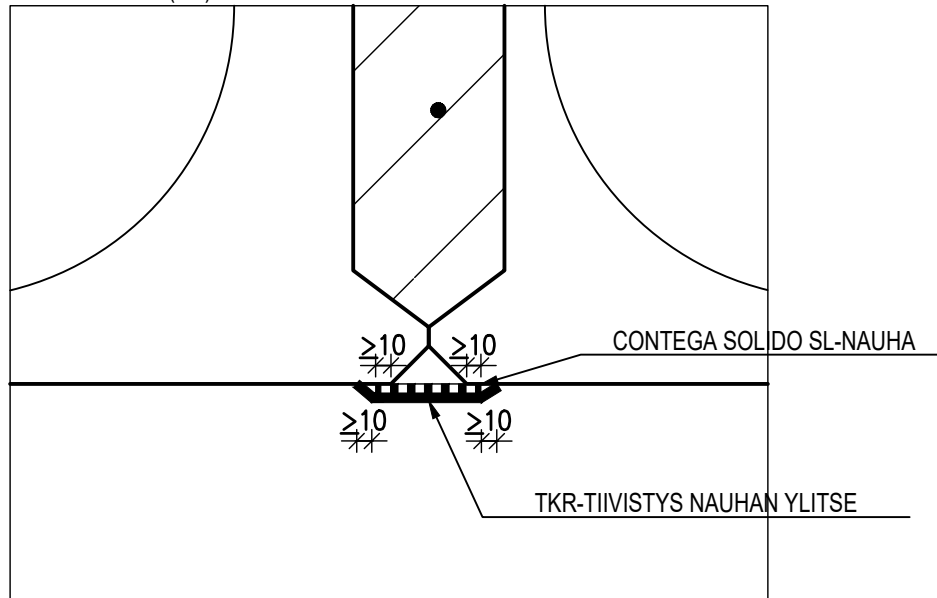
VAIHTOEHTO 2 (1:2)
