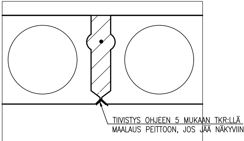
VAIHTOEHTO 1(1:5)
