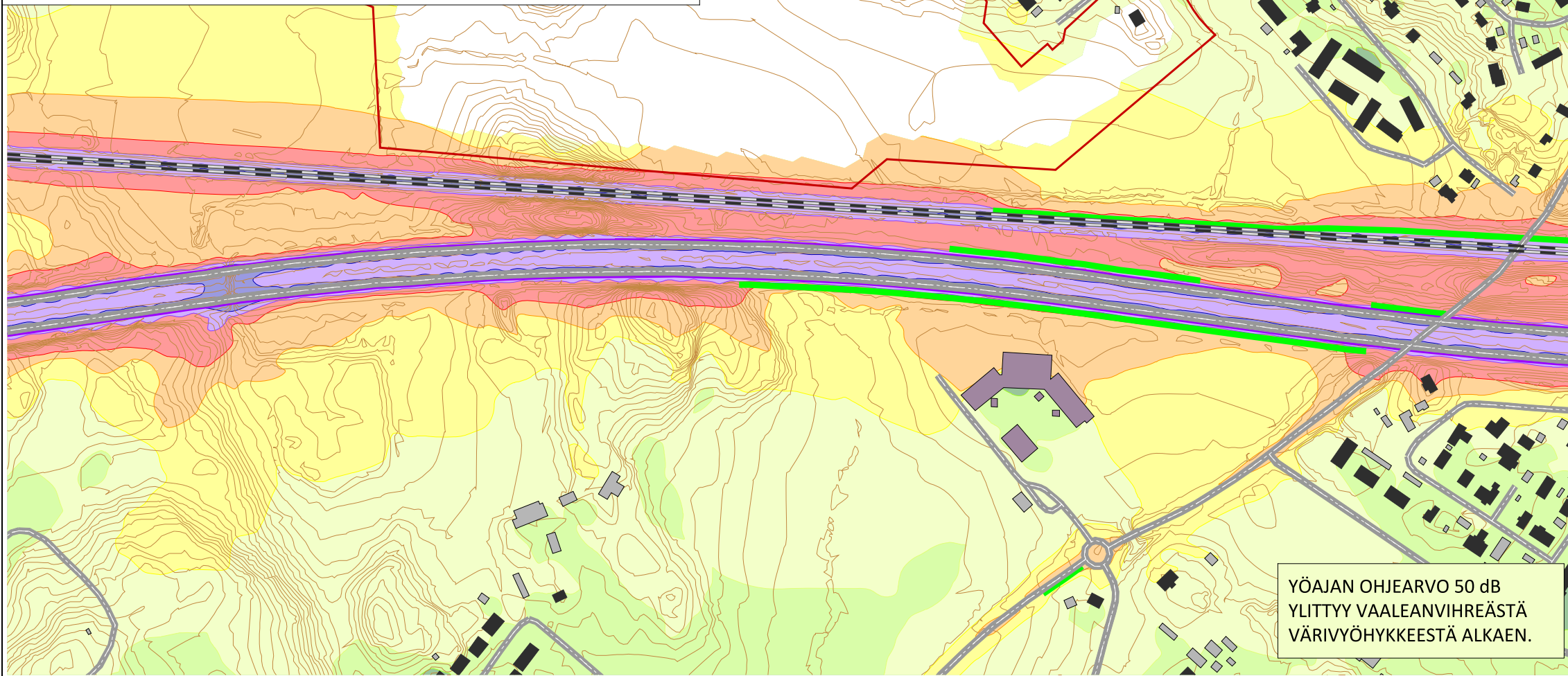
b) Yöaikaiset melutasot ennustetilanteessa nykyisellä melusuojauksella.
