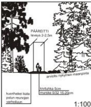
TYYPPIPOIKKILEIKKAUS A-A
