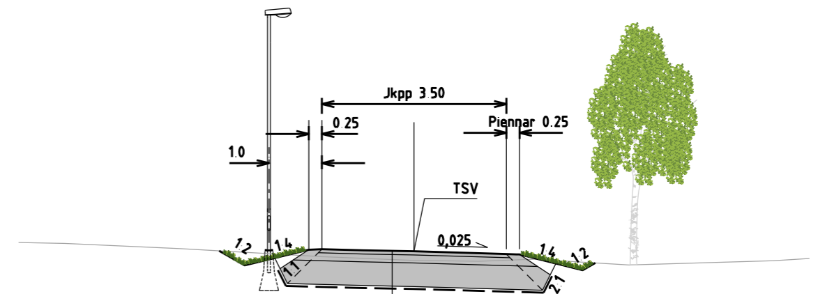
Tyypipoikkileikkaus 1:100 Esim. Paalu 20
